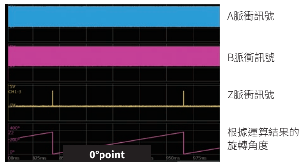
PWM波形和旋轉角度的記錄圖
