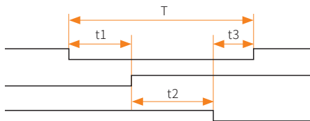
測量波形和想要求出的時間差
