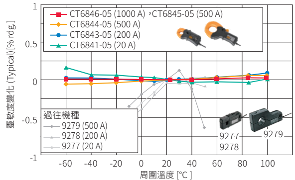
高精度感測器 勾式 根據溫度靈敏度產生變化
