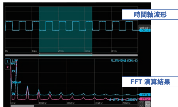
時間軸 + FFT 演算畫面
