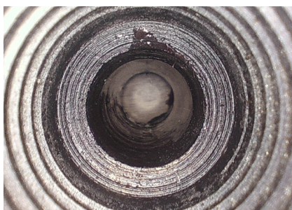
空壓機螺孔
